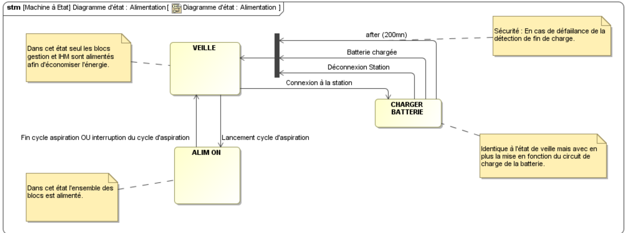
Diagramme d'états du bloc alimentation :
